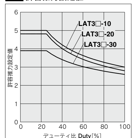
図4 許容推力設定値
