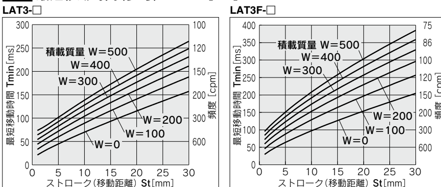
図3 最短移動時間(参考)：Tmin[ms]
