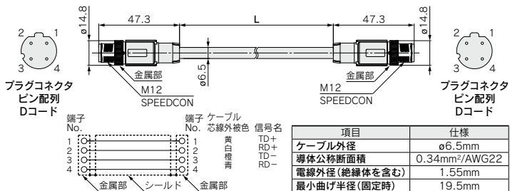
結線図(ストレートケーブル)
