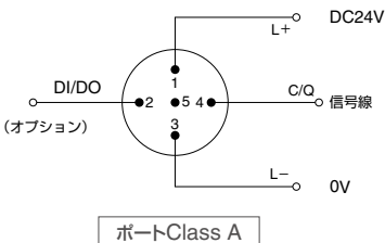
ポートClass A
