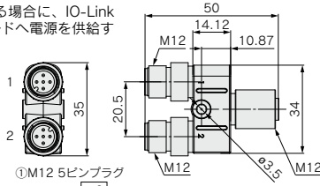
①M12 5ピンプラグ
