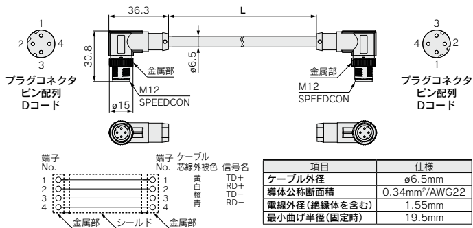
結線図(ストレートケーブル)
