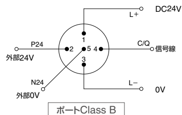
ポートClass B
